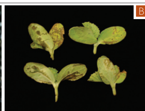
Figura 3. Típicas lesiones de BFB en A) Cotiledones de sandía y B) cotiledones de Melón.
